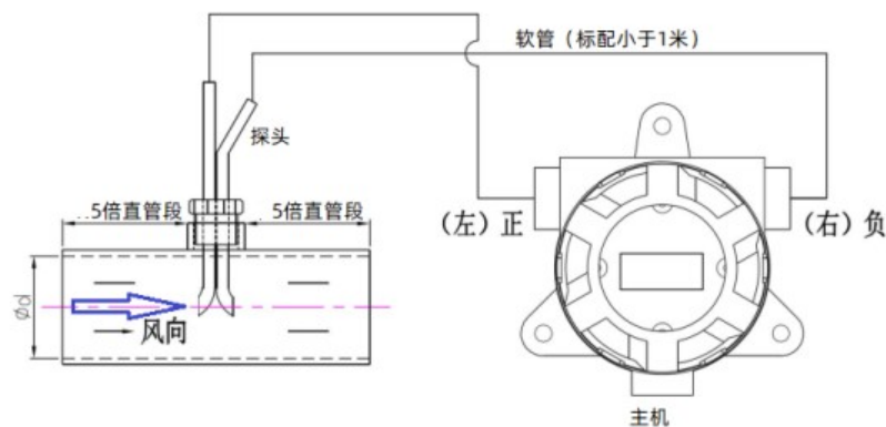
分体式安装示意图
