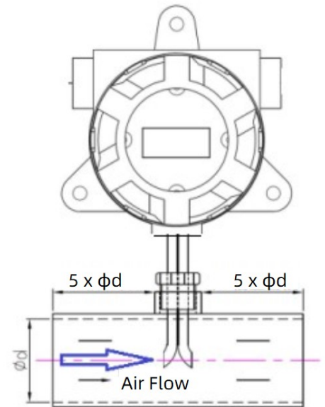
一体式安装示意图
